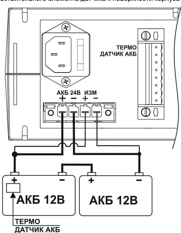
Рисунок 5 - Схема соединения аккумуляторов
